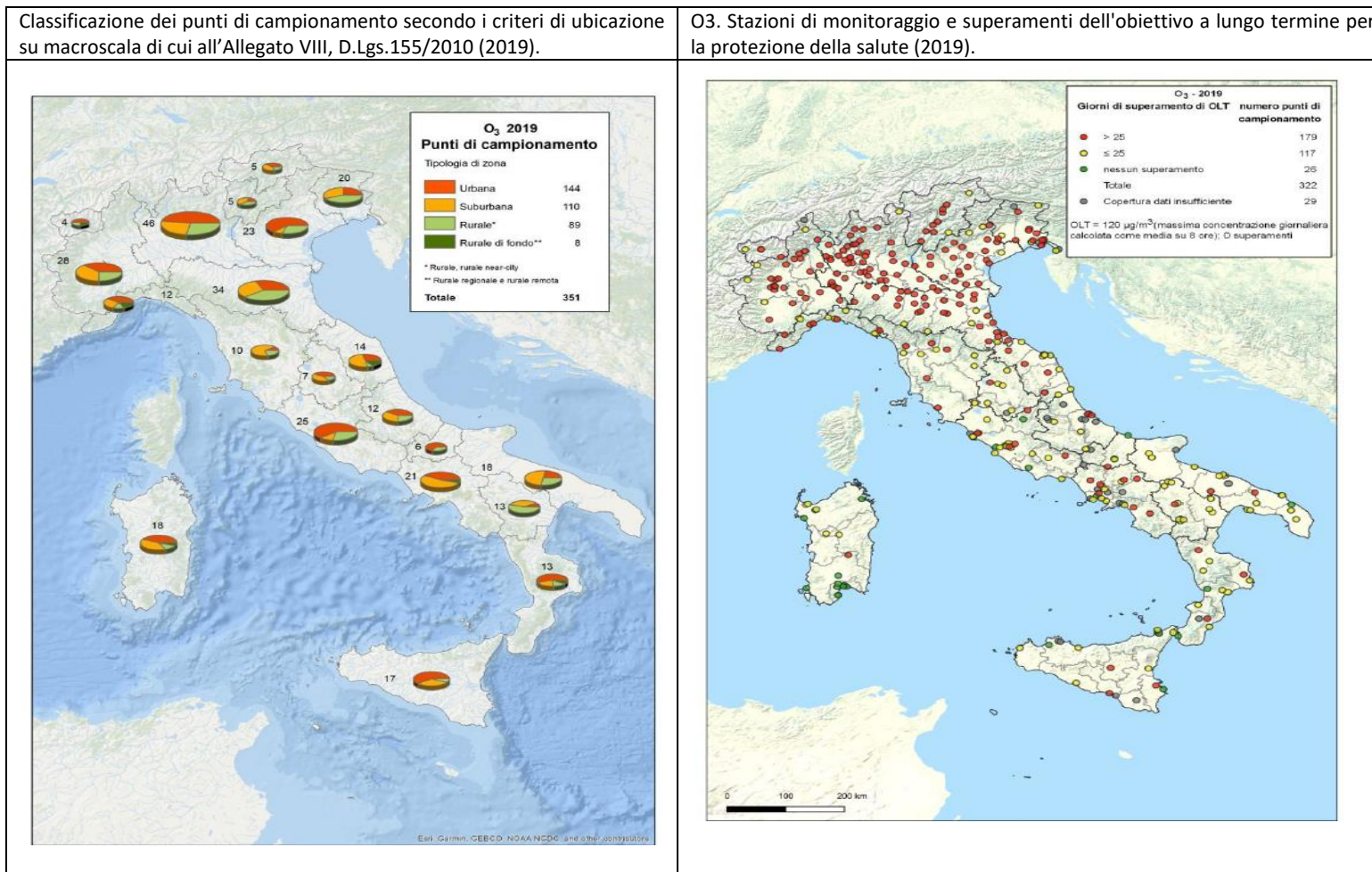
Figura 27. O 3 . Stazione di monitoraggio e superamenti dell'obiettivo a lungo termine
